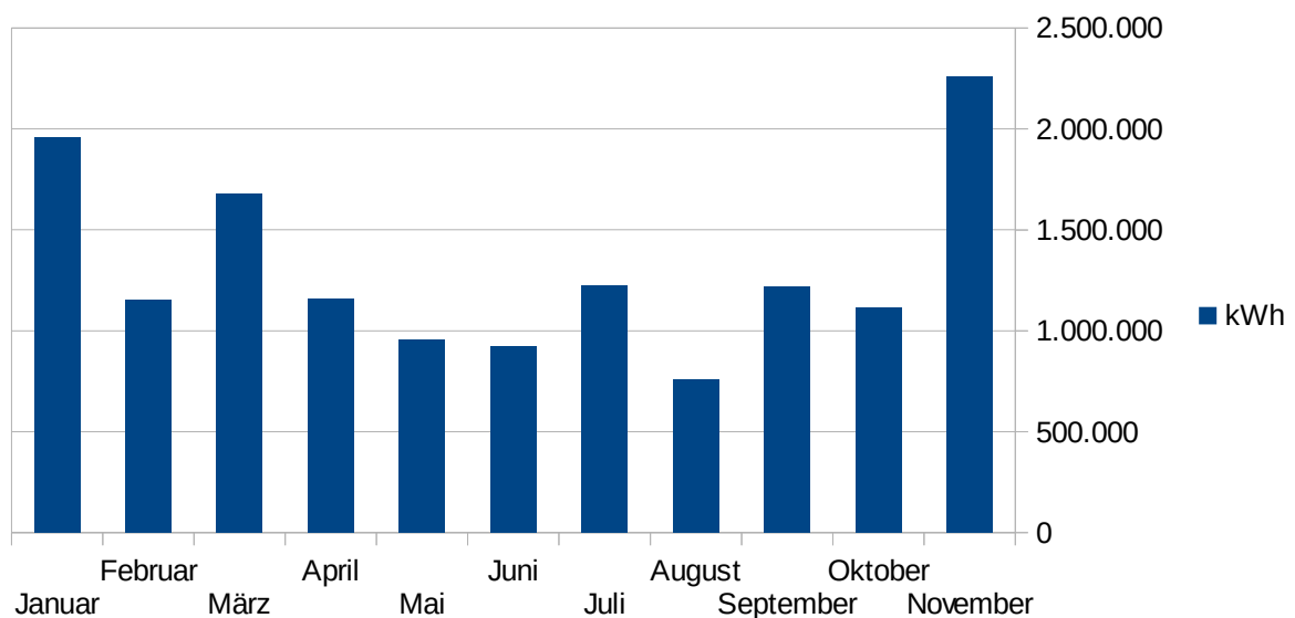
Energieertrag Jahresverlauf
