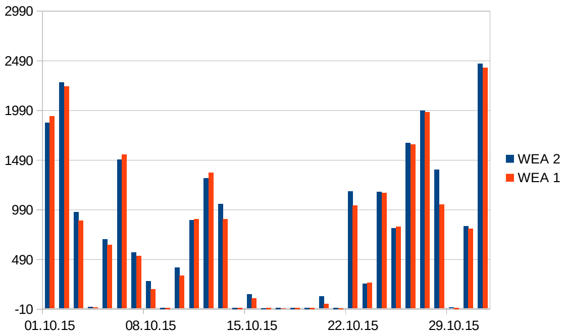
Durchschnittliche Anlagenleistung in kW
