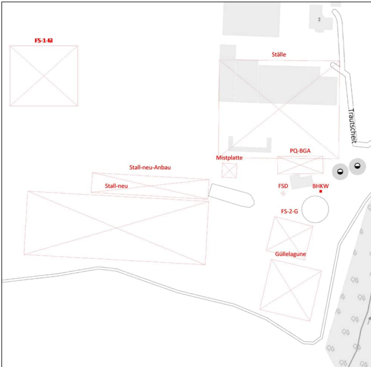
Abbildung 2: Quellenplan der Anlage im geplanten Zustand
