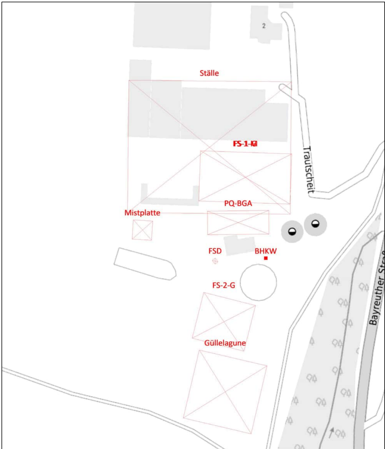
Abbildung 1: Quellenplan der Anlage im aktuellen Zustand
