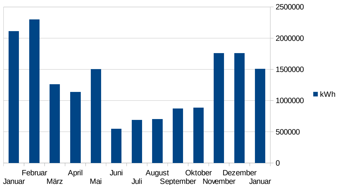
Energieertrag Jahresverlauf
